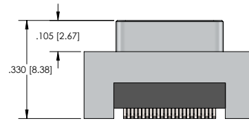
PLUG (PINS)
